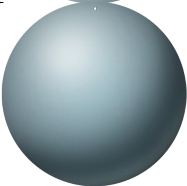
Uranus
