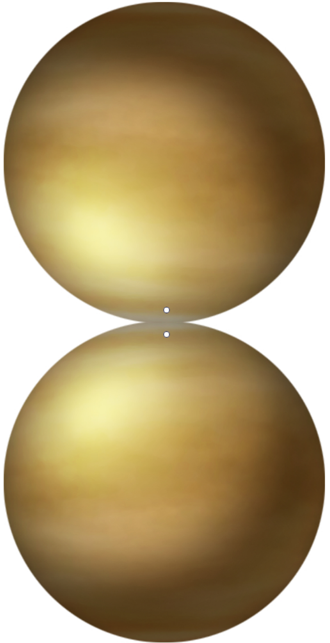
Venus
